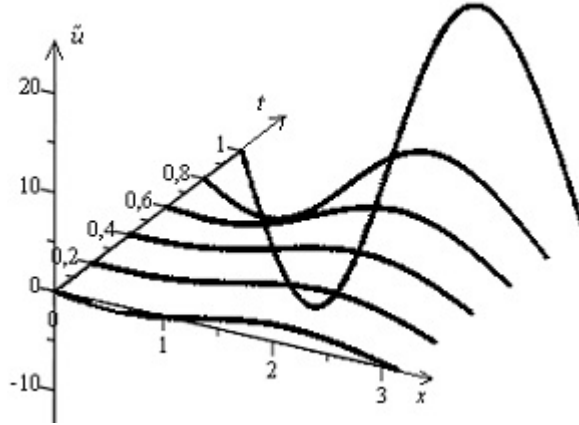
Рис. 3. График приближенного решения задачи (21)–(23)
